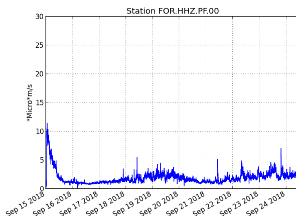
Figure 1 : Evolution du RSAM (indicateur du trémor volcanique et de l'intensité de l'éruption) entre 04h00 (00h UTC) le 15 septembre et 16h00 (12h00 UTC) le 24 septembre sur la station sismique FOR, localisée à proximité du cratère Château Fort (2000 m d'altitude sur le flanc sud-est du cône terminal).
