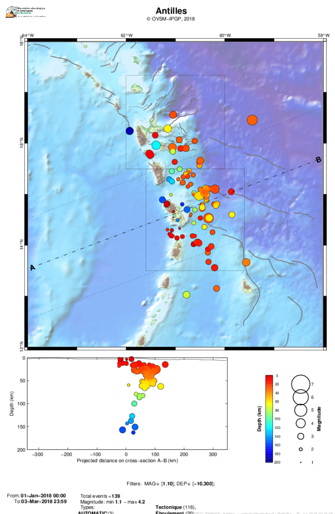
Figure 1. Carte des épicentres (partie supérieure de la figure) et représentation verticale suivant le profil A-B des mois de janvier, février et mars 2018 correspondant aux séismes enregistrés et localisés par l'OVSM-IPGP. Pour chaque séisme, la couleur correspond à la profondeur et le diamètre est proportionnel à la magnitude calculée par l'OVSM-IPGP. Traits noirs = failles principales connues (d'après Feuillet et al. 2000).
