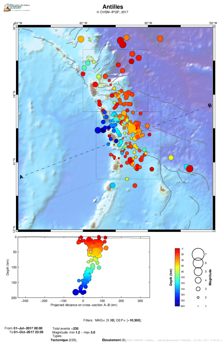
Figure 1. Carte des épicentres (partie supérieure de la figure) et représentation verticale suivant le profil A-B des mois de juillet, août et septembre 2017 correspondant aux séismes enregistrés et localisés par l'OVSM-IPGP. Pour chaque séisme, la couleur correspond à la profondeur et le diamètre est proportionnel à la magnitude calculée par l'OVSM-IPGP. Traits noirs = failles principales connues (d'après Feuillet et al. 2000).
