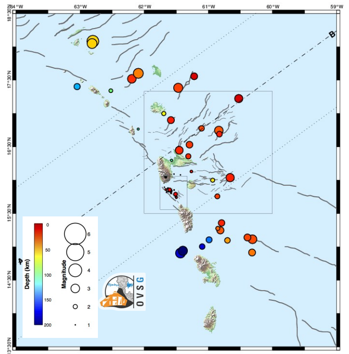
Figure 1. Carte des épicentres du mois d'août 2017 correspondant aux séismes enregistrés et localisés par l'OVSG-IPGP autour de la Guadeloupe.
