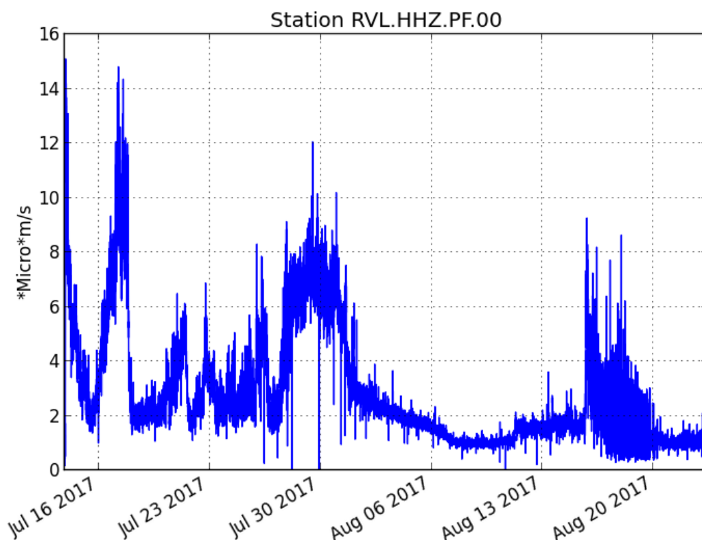
Figure 1 : Evolution du RSAM (indicateur du trémor volcanique et de l'intensité de l'éruption) entre 00h00 (20h UTC) le 14 juillet et 15h00 (11h00 UTC) le 23 août sur la station sismique de RVL, localisée sur le flanc sud du volcan.
