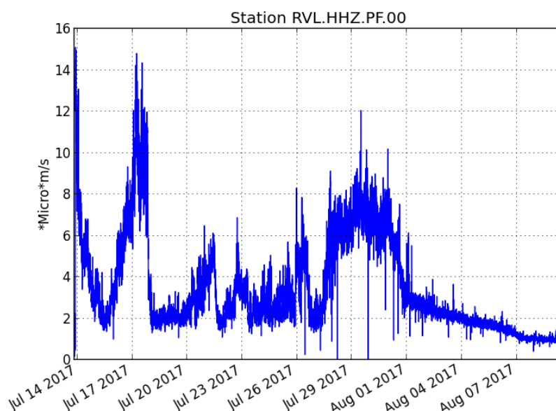
Figure 1 : Evolution du RSAM (indicateur du trémor volcanique et de l'intensité de l'éruption) entre 00h00 (20h UTC) le 14 juillet et 16h30 (12h30 UTC) le 9 août sur la station sismique de RVL, localisée sur le flanc sud du volcan.
