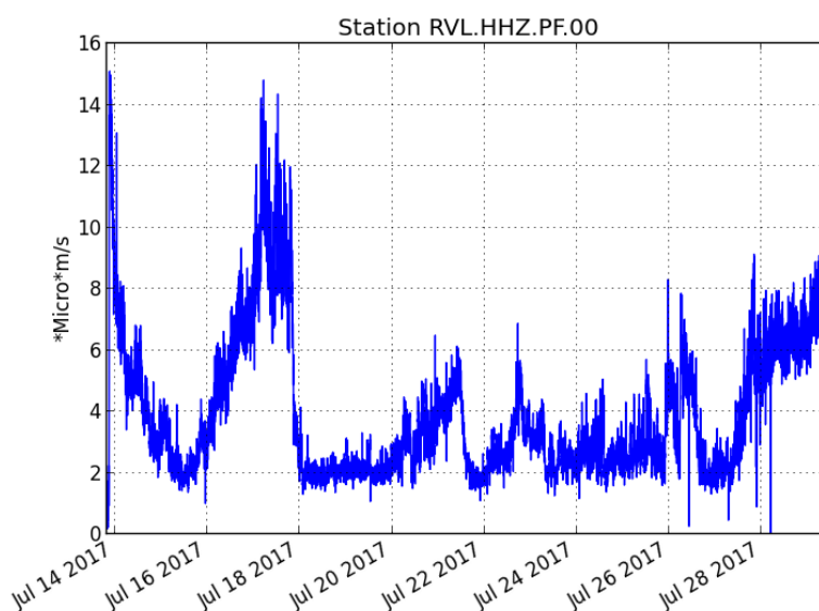
Figure 1 : Evolution du RSAM (indicateur du trémor volcanique et de l'intensité de l'éruption) entre 00h00 (20h UTC) le 14 juillet et 15h30 (11h30 UTC) le 29 juillet sur la station sismique de RVL, localisée sur le flanc sud du volcan.
