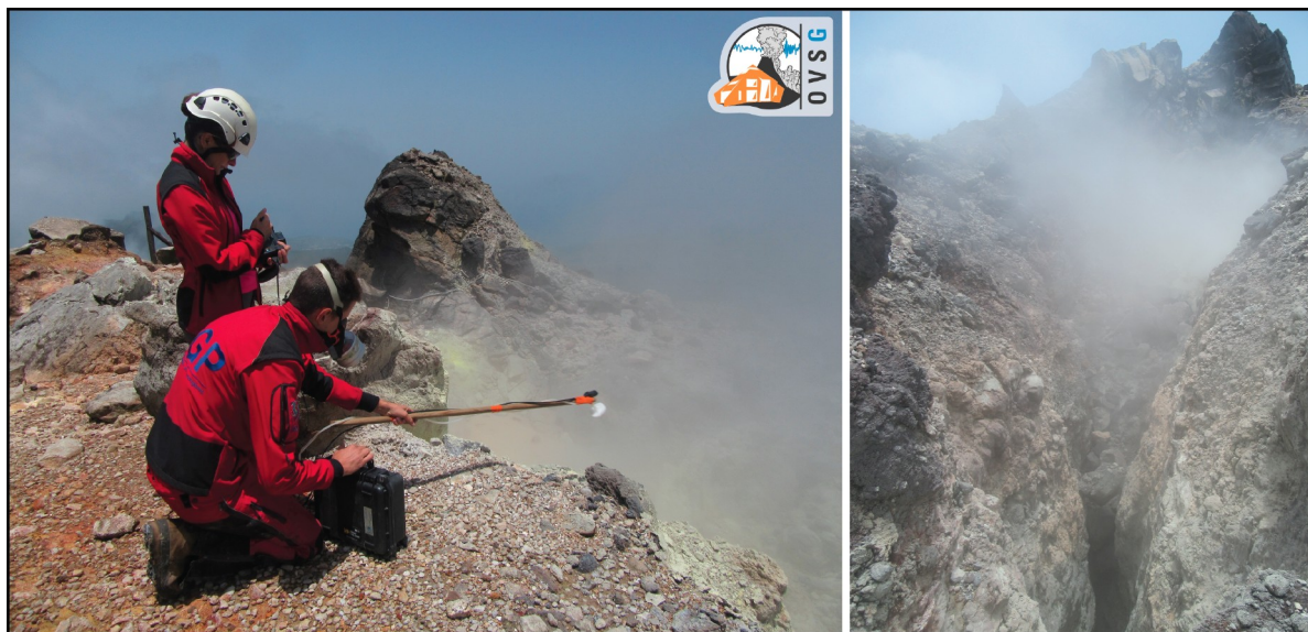
27 juin 2017. Fumerolle du Cratère Sud dans sa partie sud © C.Dessert-IPGP.
