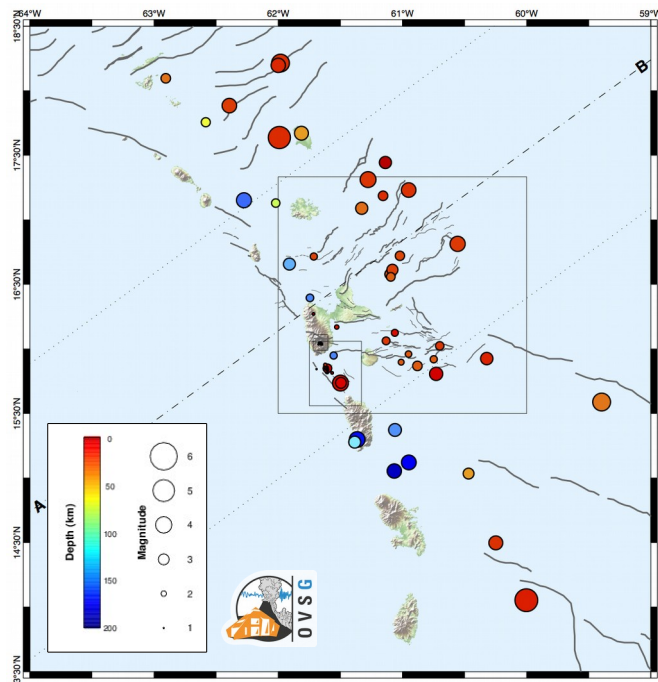
Figure 1. Carte des épicentres du mois de juin 2017 correspondant aux séismes enregistrés et localisés par l'OVSG-IPGP autour de la Guadeloupe.
