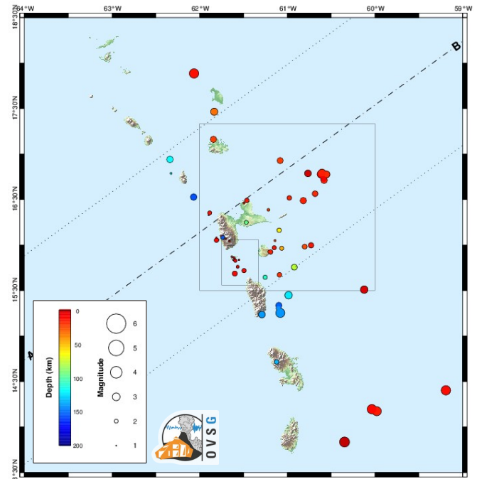
Figure 1. Carte des épïcêtres du mois de janvier 2017 correspondant aux séismes enregistrés et localisés par l'OVSG-IPGP autour de la Guadeloupe. Traits noirs = failles principales connues (d'après Feuillet et al. 2000).
