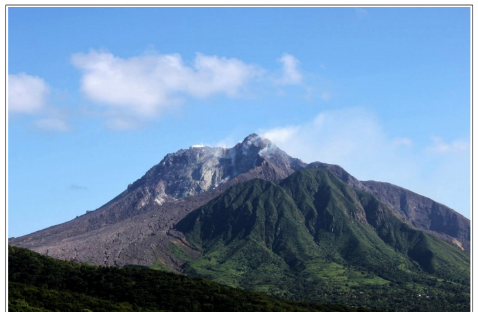
Photo 1. Volcan Soufrière Hills le 12 janvier 2017 © MVO. Les conditions météorologiques clémentes permettent parfois d'observer les fumeroles du dôme, sans pour cela attester d'une augmentation de l'activité volcanique.
