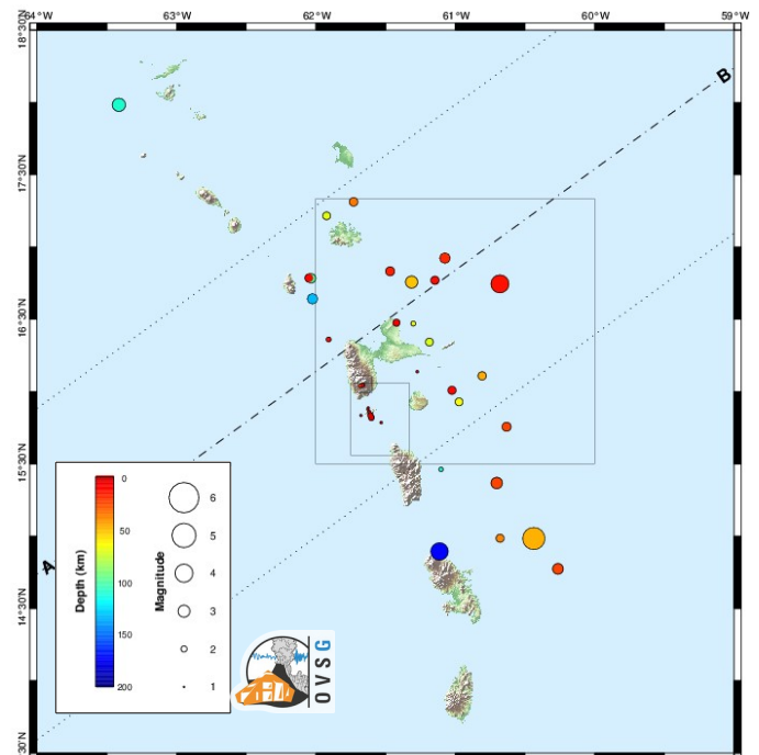
Figure 1. Carte des épacentres du mois de décembre 2016 correspondant aux séismes enregistrés et localisés par l'OVSG-IPGP autour de la Guadeloupe. Traits noirs = failles principales connues (d'après Feuillet et al. 2000).
