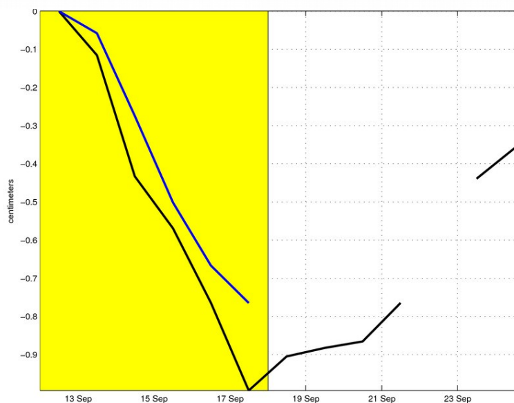
Figure 2: Illustration de la déformation sommitale depuis le début de l'éruption du 11-18 Septembre 2016 (en jaune). Est ici représentée une ligne de base (distance entre deux récepteurs GPS) traversant le cratère Dolomieu d'est en ouest (en noir les données brutes, en bleu les données lissées sur une semaine). Une hausse est synonyme d'élongation et donc de gonflement du volcan.
