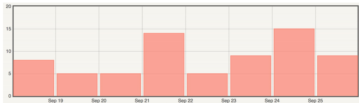
Figure 1: Bilan de la sismicité volcano-tectonique superficielle au Piton de la Fournaise du 18 au 25 Septembre (19:00 heure locale) 2016.
