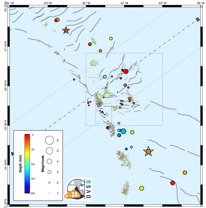
Figure 1. Carte des épicentres du mois de juin 2016 correspondant aux séismes enregistrés et localisés par l'OVSG-IPGP autour de la Guadeloupe. Traits noirs = failles principales connues (d'après Feuillet et al. 2000) ; Etoile = séisme ressenti.
