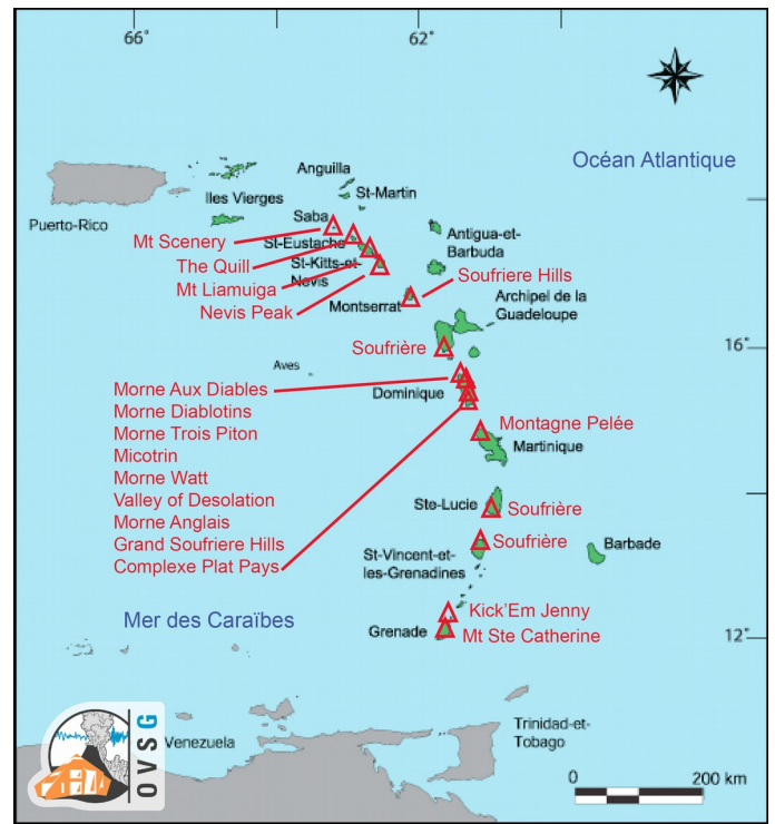
Figure 2. Carte des volcans actifs de l'arc des Petites Antilles.
