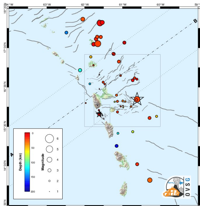
Figure 1. Carte des épacentres du mois de mai 2016 correspondant aux séismes enregistrés et localisés par l'OVSG-IPGP autour de la Guadeloupe. Traits noirs = failles principales connues (d'après Feuillet et al. 2000) ; Etoile = séisme ressenti.
