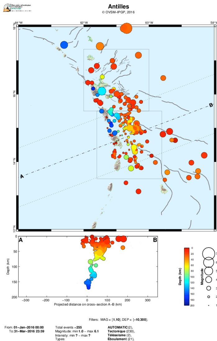
Figure 1. Carte des épicentres (partie supérieure de la figure) et représentation verticale suivant le profil A-B des mois de janvier, février et mars 2016 correspondant aux séismes enregistrés et localisés par l'OVSM-IPGP. Pour chaque séisme, la couleur correspond à la profondeur et le diamètre est proportionnel à la magnitude calculée par l'OVSM-IPGP. Traits noirs = failles principales connues (d'après Feuillet et al. 2000).
