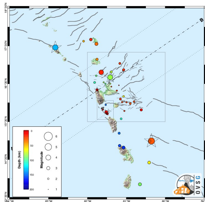
Figure 1. Carte des épacentres des séismes enregistrés et localisés par l'OVSG-IPGP autour de la Guadeloupe. Traits noirs = failles principales connues (d'après Feuillet et al. 2000) ; Etoile = séisme ressenti.
