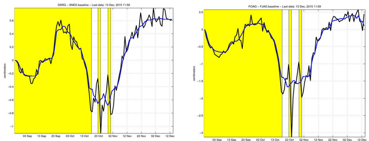
Figure 2 : Illustration de la déformation. Sont ici représentées deux lignes de base (distance entre deux GPS) au sommet (à gauche) et à la base du cône sommitale (à droite).
