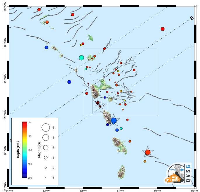
Figure 1. Carte des épacentres du mois de novembre 2015 correspondant aux séismes enregistrés et localisés par l'OVSG-IPGP autour de la Guadeloupe. Traits noirs = failles principales connues (d'après Feuillet et al. 2000).
