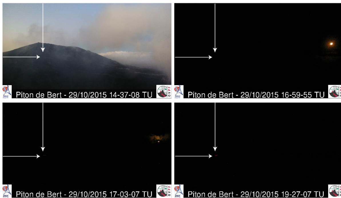
Figure 2 : Evidence de la reprise de l'activité dans le cône visible à partir de 20H locale (17H TU)
