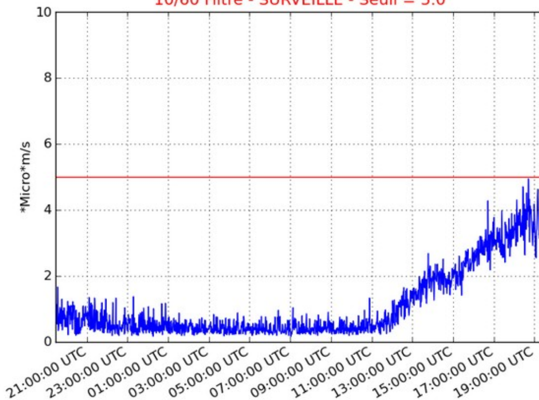
Figure 1 : Intensité à la station Rivals à 23H30
