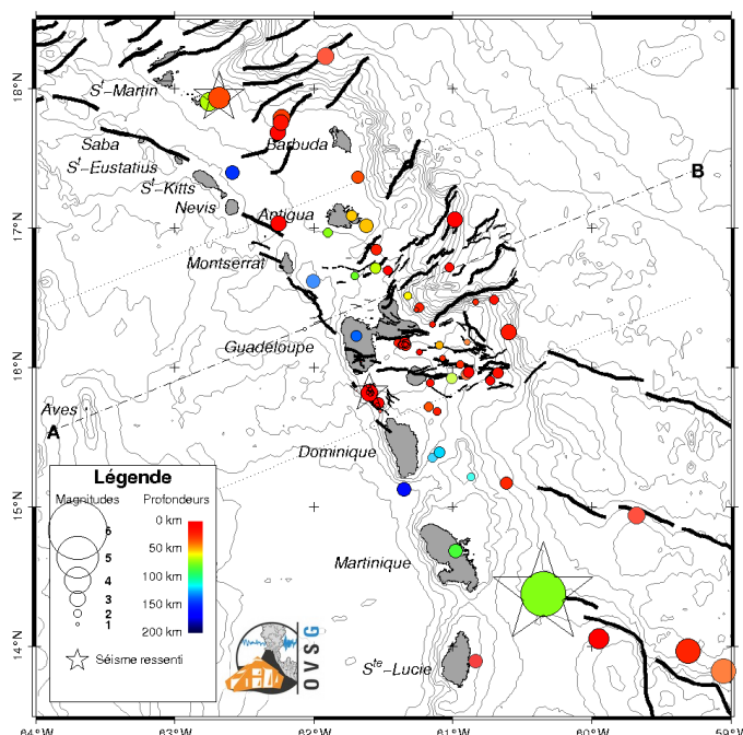
Figure 1. Carte des épïcêtres du mois d'août 2015 correspondant aux séismes enregistrés et localisés par l'OVSG-IPGP autour de la Guadeloupe. Traits noirs = failles principales connues (d'après Feuillet et al. 2000).
