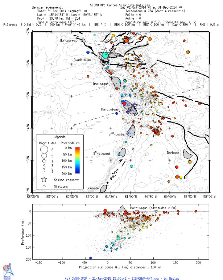
Figure 1. Carte des épicentres (partie supérieure de la figure) et représentation verticale suivant le profil A-B des mois d'octobre, novembre et décembre 2014 correspondant aux séismes enregistrés et localisés par l'OVSM-IPGP. Pour chaque séisme, la couleur correspond à la profondeur et le diamètre est proportionnel à la magnitude calculée par l'OVSM-IPGP. Étoile : séisme ressenti (Martinique et/ou Guadeloupe). Traits noirs = failles principales connues (d'après Feuillet et al. 2000).
