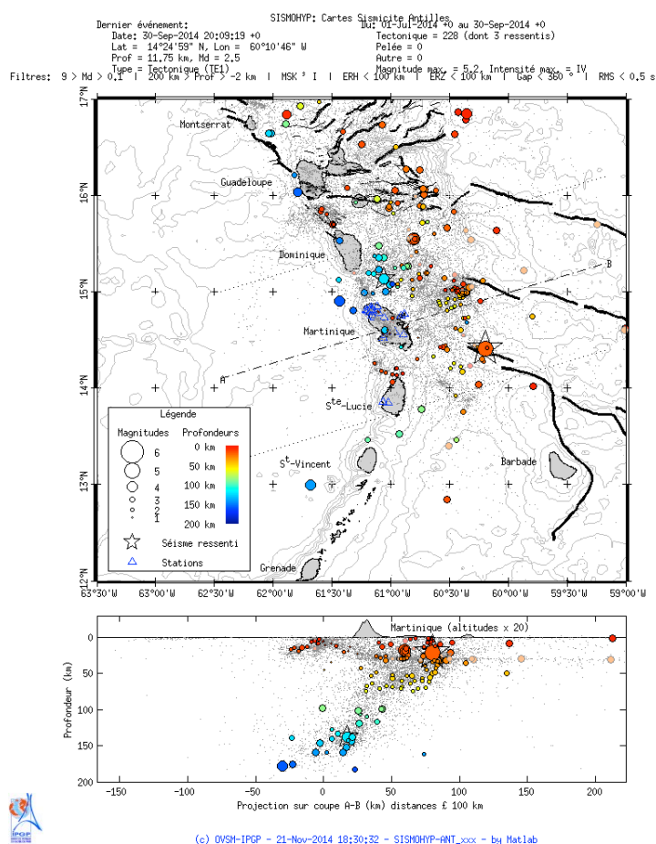
Figure 1. Carte des épicentres (partie supérieure de la figure) et représentation verticale suivant le profil A-B des mois de juillet, août et septembre 2014 correspondant aux séismes enregistrés et localisés par l'OVSM-IPGP. Pour chaque séisme, la couleur correspond à la profondeur et le diamètre est proportionnel à la magnitude calculée par l'OVSM-IPGP. Étoile : séisme ressenti. Traits noirs = failles principales connues (d'après Feuillet et al. 2000).
