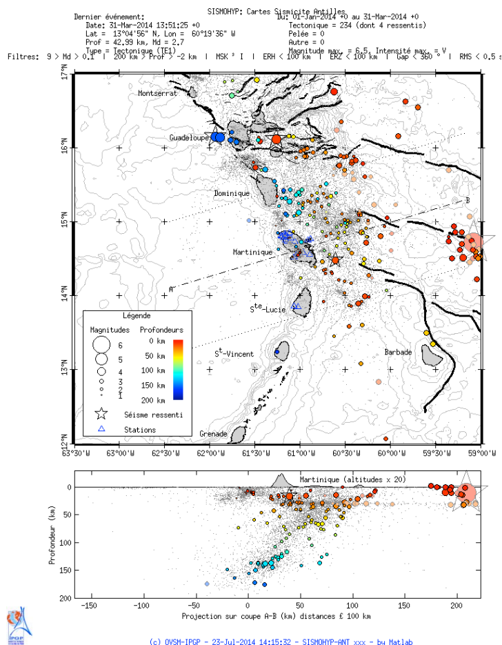
Figure 1. Carte des épicentres (partie supérieure de la figure) et représentation verticale suivant le profil A-B des mois de janvier, février et mars 2014 correspondant aux séismes enregistrés et localisés par l'OVSM-IPGP. Pour chaque séisme, la couleur correspond à la profondeur et le diamètre est proportionnel à la magnitude calculée par l'OVSM-IPGP. Étoile : séisme ressenti. Traits noirs = failles principales connues (d'après Feuillet et al. 2000).
