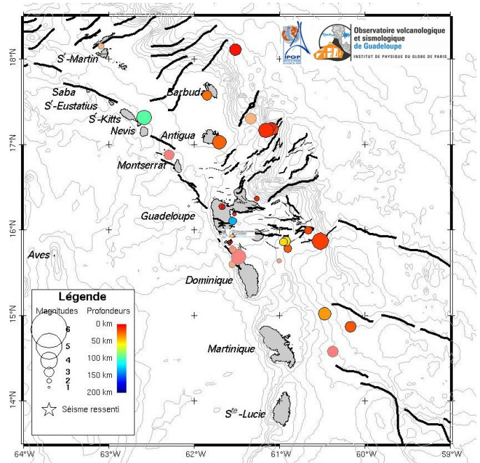
Figure 1. Carte des épïcêtres du mois de juin 2013 correspondant aux séismes enregistrés et localisés par l'OVSG-IPGP dans un rayon de 450 km autour de la Guadeloupe. Traits noirs = failles principales connues (d'après Feuillet et al. 2000).
