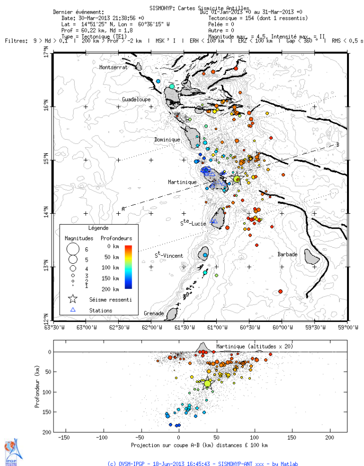
Figure 1. Carte des épicentres (partie supérieure de la figure) et représentation verticale suivant le profil A-B des mois de janvier, février et mars 2013 correspondant aux séismes enregistrés et localisés par l'OVSM-IPGP. Pour chaque séisme, la couleur correspond à la profondeur et le diamètre est proportionnel à la magnitude calculée par l'OVSM-IPGP. Étoile : séisme ressenti. Traits noirs = failles principales connues (d'après Feuillet et al. 2000).
