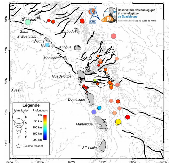
Figure 1. Carte des épicentres du mois de janvier 2013
