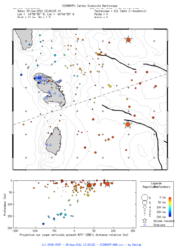
Figure 1. Carte des épicentres et représentation verticale suivant le profil A-B des mois de avril, mai et juin 2011 correspondant aux séismes enregistrés et localisés par l'OVSM-IPGP. Pour chaque séisme, la couleur correspond à la profondeur et le diamètre est proportionnel à la magnitude calculée par l'OVSM-IPGP. Etoile : séisme ressenti. Traits noirs = failles principales connues (d'après Feuillet et al. 2000).
