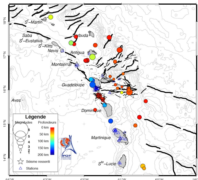
Figure 1. Carte des épocentres du mois de juin 2011 correspondant aux séismes enregistrés et localisés par l'OVSG-IPGP dans un rayon de 450 km autour de la Guadeloupe. Traits noirs = failles principales connues (d'après Feuillet et al. 2000).
