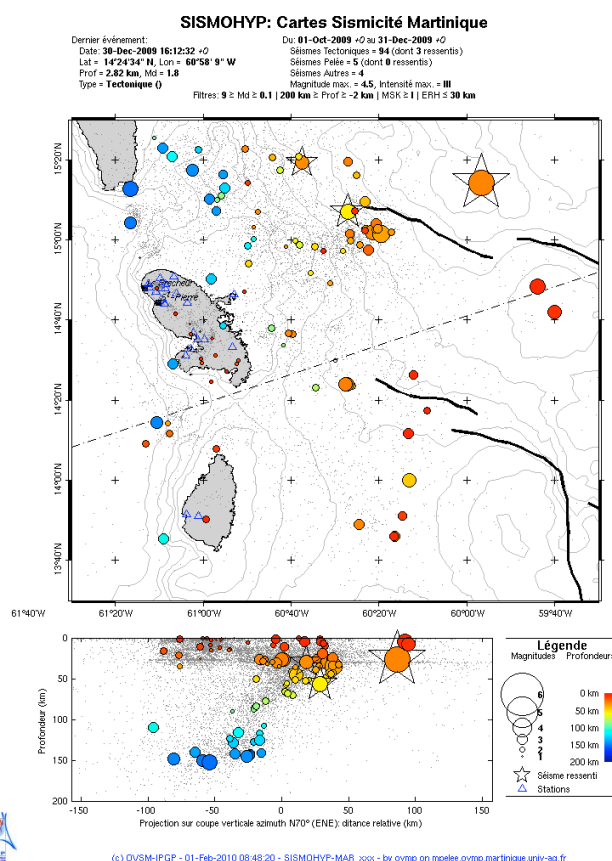
Figure 1. Carte des épencentres et représentation verticale suivant le profil A-B des mois d'octobre, novembre et décembre 2009 correspondant aux séismes enregistrés et localisés par l'OVSM-IPGP. Pour chaque séisme, la couleur correspond à la profondeur et le diamètre est proportionnel à la magnitude calculée par l'OVSM-IPGP. Etoile : séisme ressenti. Traits noirs = failles principales connues (d'après Feuillet et al. 2000).
