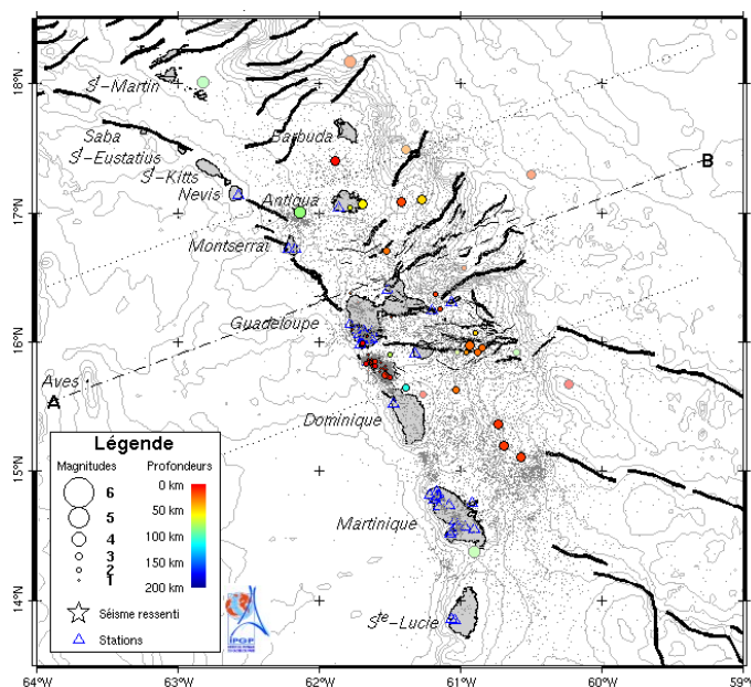
Figure 1. Carte des épicentres du mois de juin 2007 correspondant aux séismes enregistrés et localisés par l'OVSG-IPGP (voir la légende). Traits noirs = failles principales connues (d'après Feuillet, 2000), traits gris = courbes bathymétriques.
