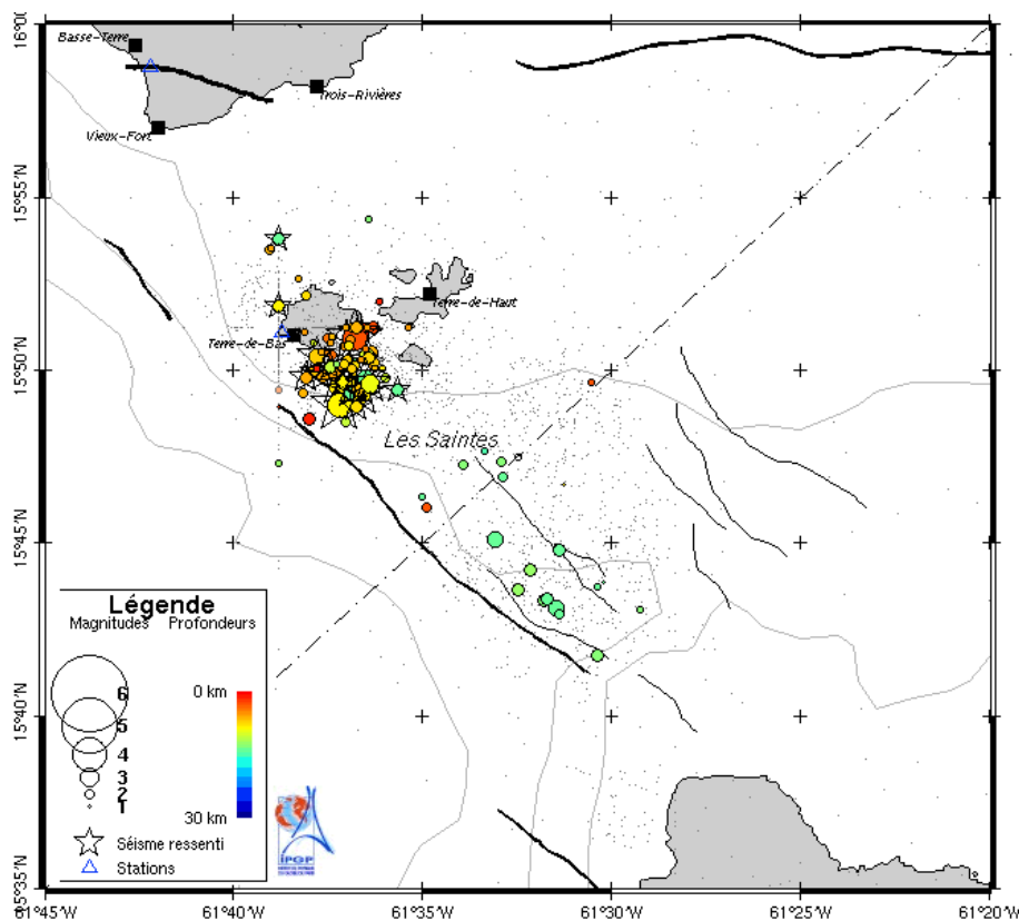
Figure 2. Localisations préliminaires des 102 plus fortes répliques du mois d'octobre 2005 : taille des symboles = magnitude, couleur = profondeur, étoiles = séisme supposé ressenti, traits noirs = failles connues, traits gris = courbes bathymétriques.
